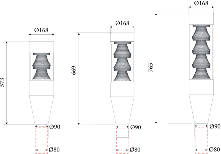
2.12. ЧЕРТЕЖ.
