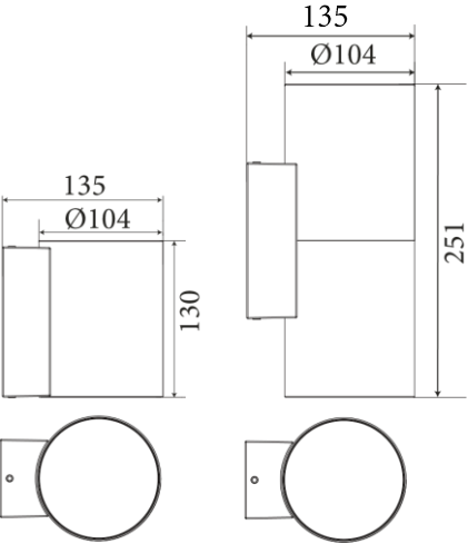
2.13. ЧЕРТЕЖ.
