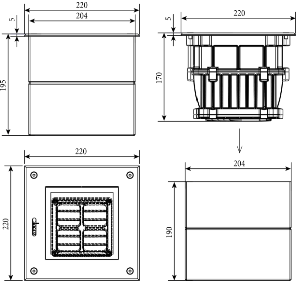
2.17. ЧЕРТЕЖ.
