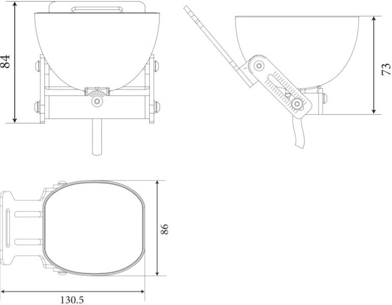
2.12. ЧЕРТЕЖ.
