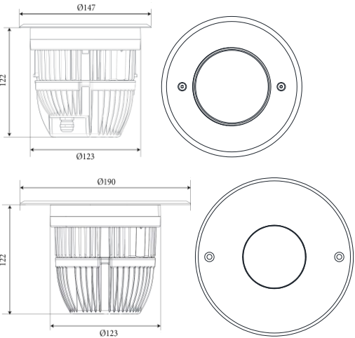
2.13. ЧЕРТЕЖ.
