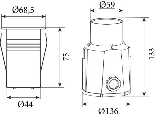
2.14. ЧЕРТЕЖ.
