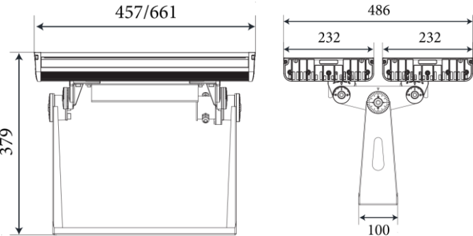
2.12. ЧЕРТЕЖ.
