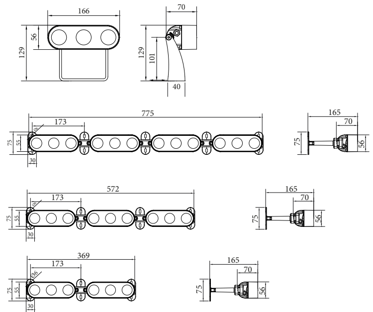
Кронштейн 1.2
