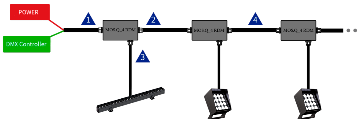
Рисунок 1. Схема подключения MOS.Q
